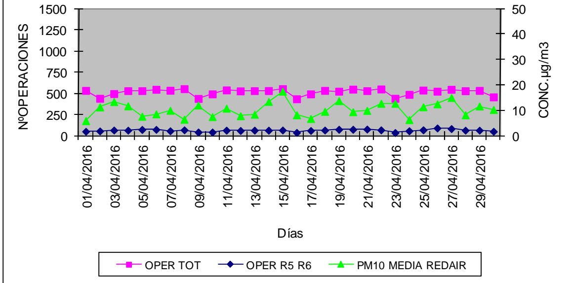
GRÁFICO COMPARATIVO: Nº OPER. TOTALES Y Nº OPER. RAMPAS 5/6 vs. CONC. PARTÍCULAS EN SUSPENSIÓN PM10 MEDIA REDAIR. ABRIL 2016.
