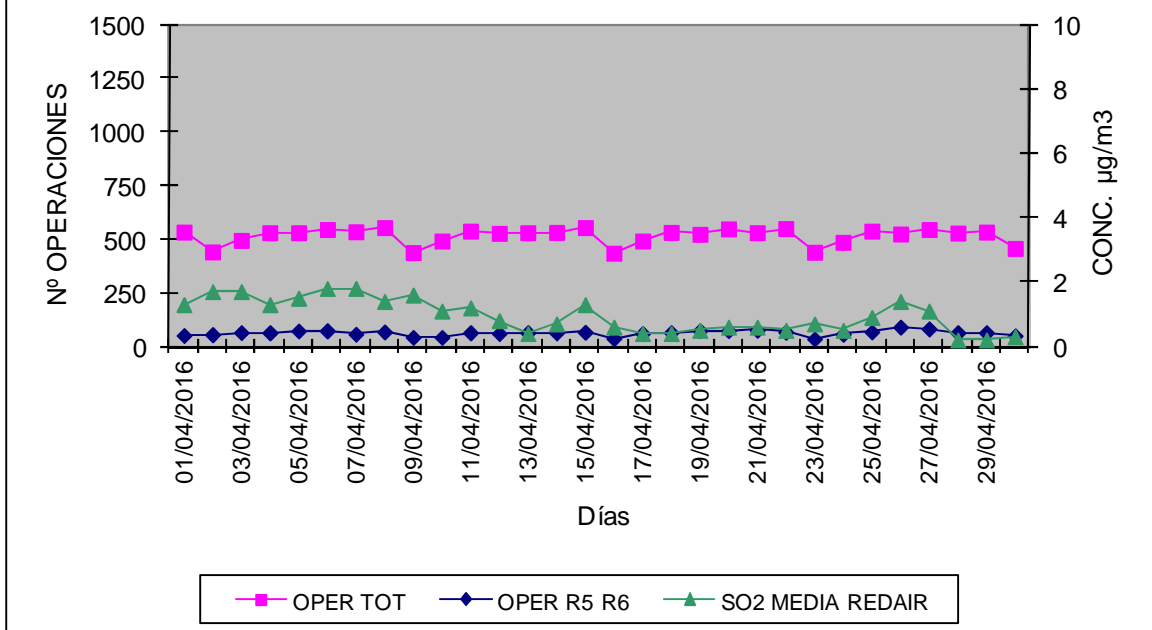
GRÁFICO COMPARATIVO: Nº OPER. TOTALES Y Nº OPER. RAMPAS 5/6 vs. CONC. SO2 MEDIA REDAIR. ABRIL 2016.
