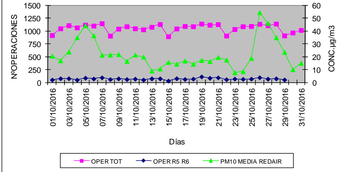
GRÁFICO COMPARATIVO: Nº OPER. TOTALES Y Nº OPER. RAMPAS 5/6 vs. CONC. PARTÍCULAS EN SUSPENSIÓN PM10 MEDIA REDAIR. OCTUBRE 2016.
