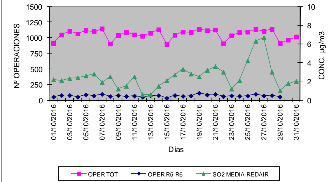
GRÁFICO COMPARATIVO: Nº OPER. TOTALES Y Nº OPER. RAMPAS 5/6 vs. CONC. SO2 MEDIA REDAIR. OCTUBRE 2016.
