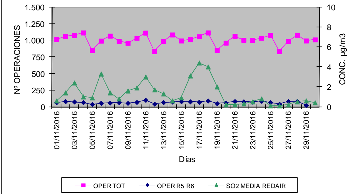
GRÁFICO COMPARATIVO: Nº OPER. TOTALES Y Nº OPER. RAMPAS 5/6 vs. CONC. SO2 MEDIA REDAIR. NOVIEMBRE 2016.
