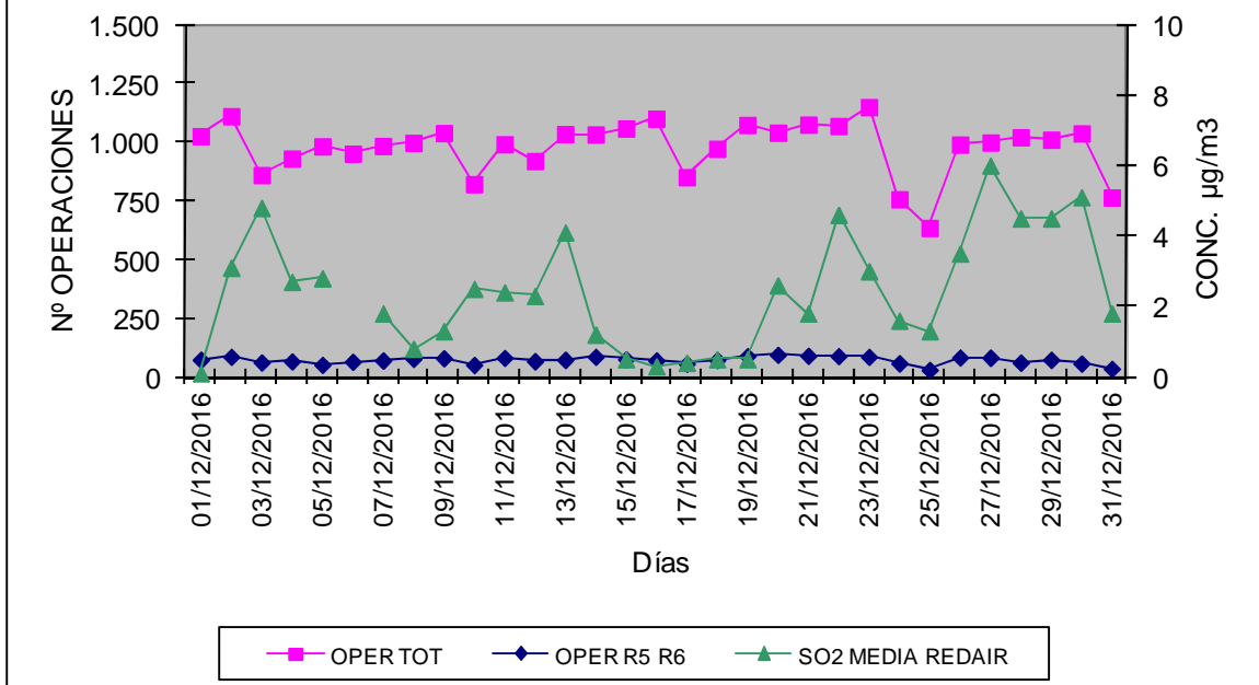
GRÁFICO COMPARATIVO: Nº OPER. TOTALES Y Nº OPER. RAMPAS 5/6 vs. CONC. SO2 MEDIA REDAIR. DICIEMBRE 2016.
