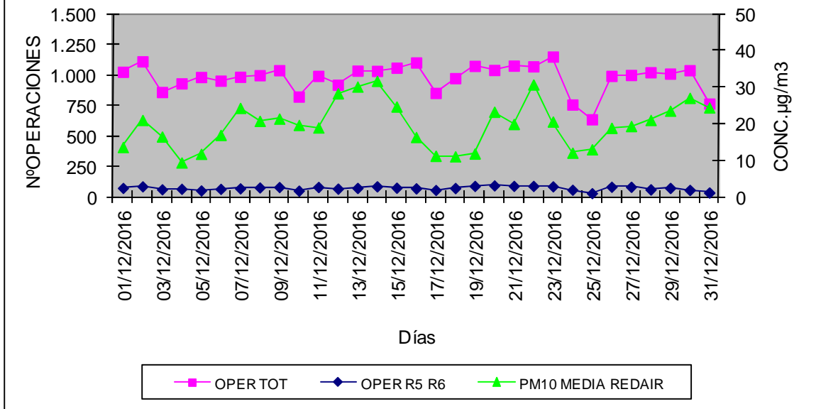
GRÁFICO COMPARATIVO: Nº OPER. TOTALES Y Nº OPER. RAMPAS 5/6 vs. CONC. PARTÍCULAS EN SUSPENSIÓN PM10 MEDIA REDAIR. DICIEMBRE 2016.
