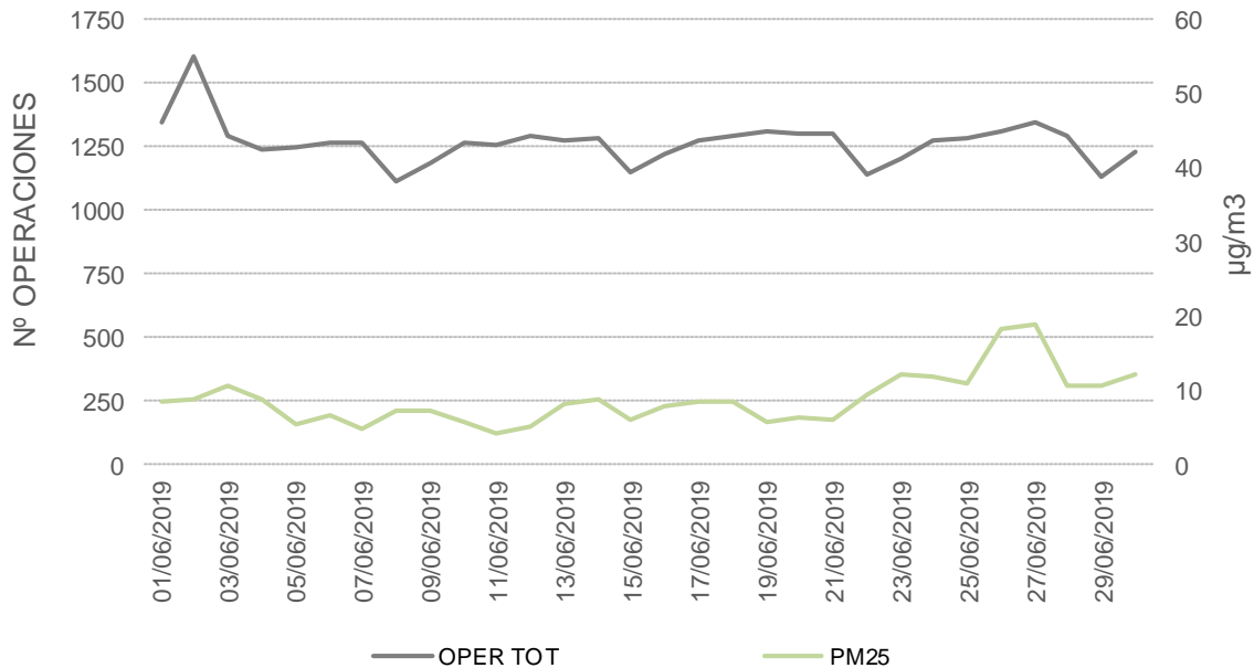
Nº OPER. TOTALES vs. CONC. PM2,5 MEDIA REDAIR.
