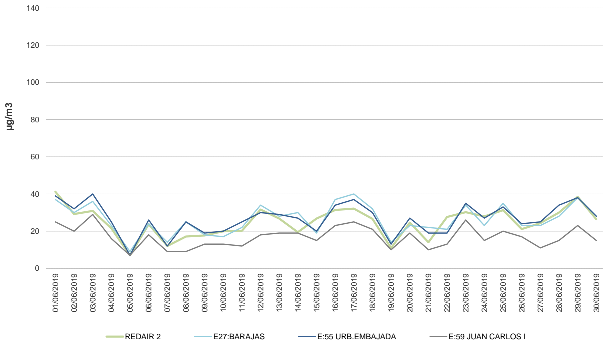
GRÁFICO COMPARATIVO DE VALORES MEDIOS DIARIOS NO2: ESTACIONES PRÓXIMAS DEL AYUNTAMIENTO DE MADRID vs. ESTACIÓN REDAIR 2. FEBRERO 2019
